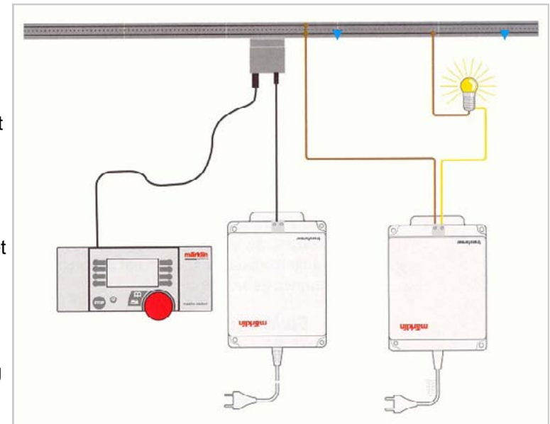
Eenvoudige constructie van een spoorbezetsmelder.
